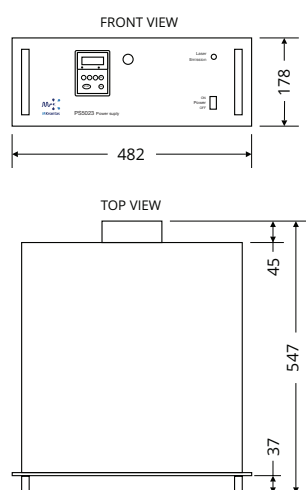
Fig. 1. Dimensions
